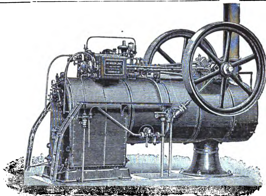
1. Полулокомобиль отъ 3 до 60 силъ.
